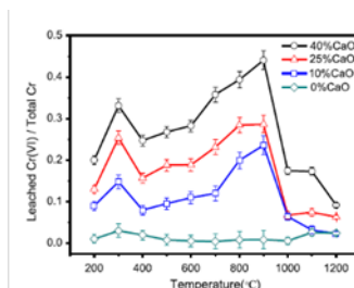
Fig.6: Cr(VI) uitlogingscurve<3>
