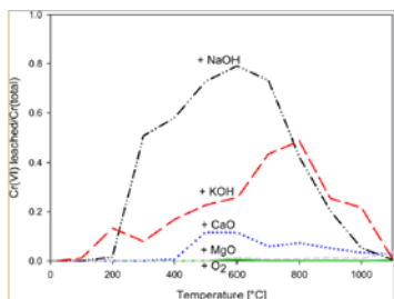
Fig. 5: Percentage uitloging Cr(III) als Cr(VI)->
